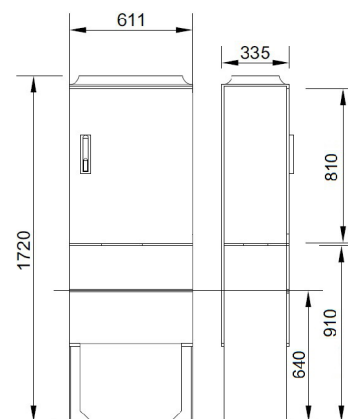
Dimensions armoire de commande (mm)
