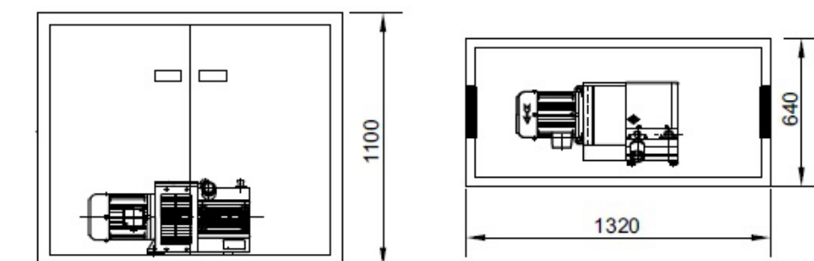
Dimensions armoire de commande (mm)
